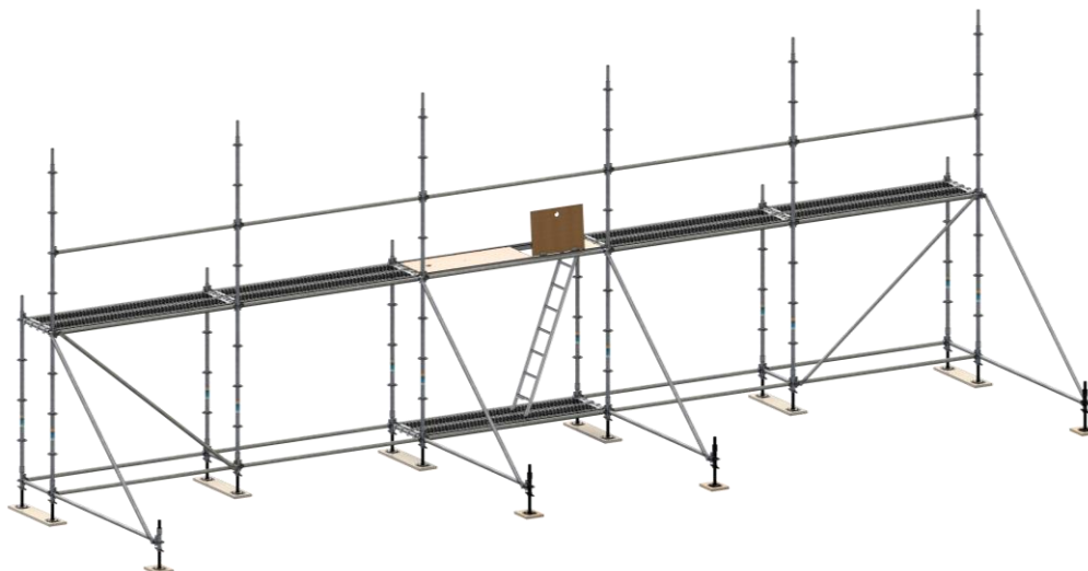
Figure 8.9 : Exemple de dispositif anti basculement temporaire.
