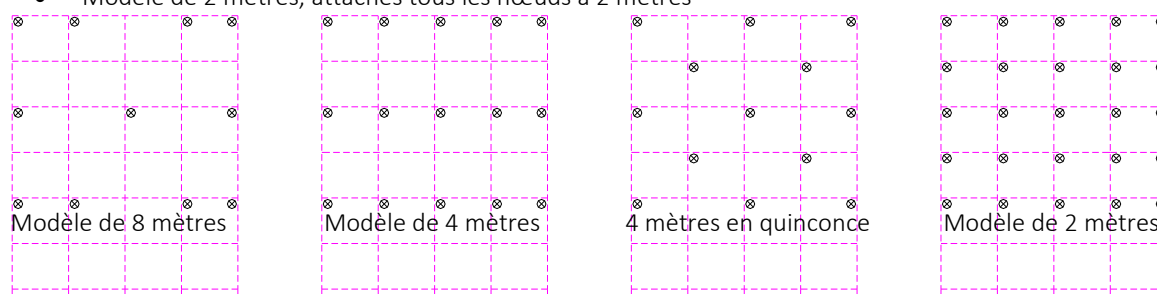
Figure 6.5 : Modèle d'ancrage
