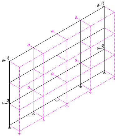
Figure 6.6 : Ancres en V
