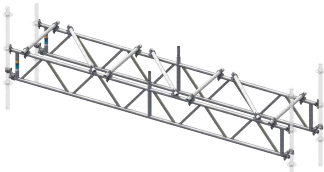
Figure 4.2 : Diagonale de deux poutres à treillis
