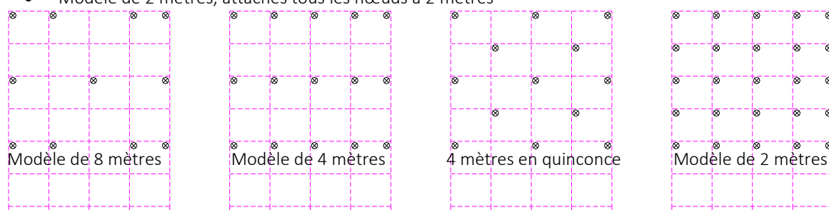
Figure 6.5 : Modèle d'ancrage
