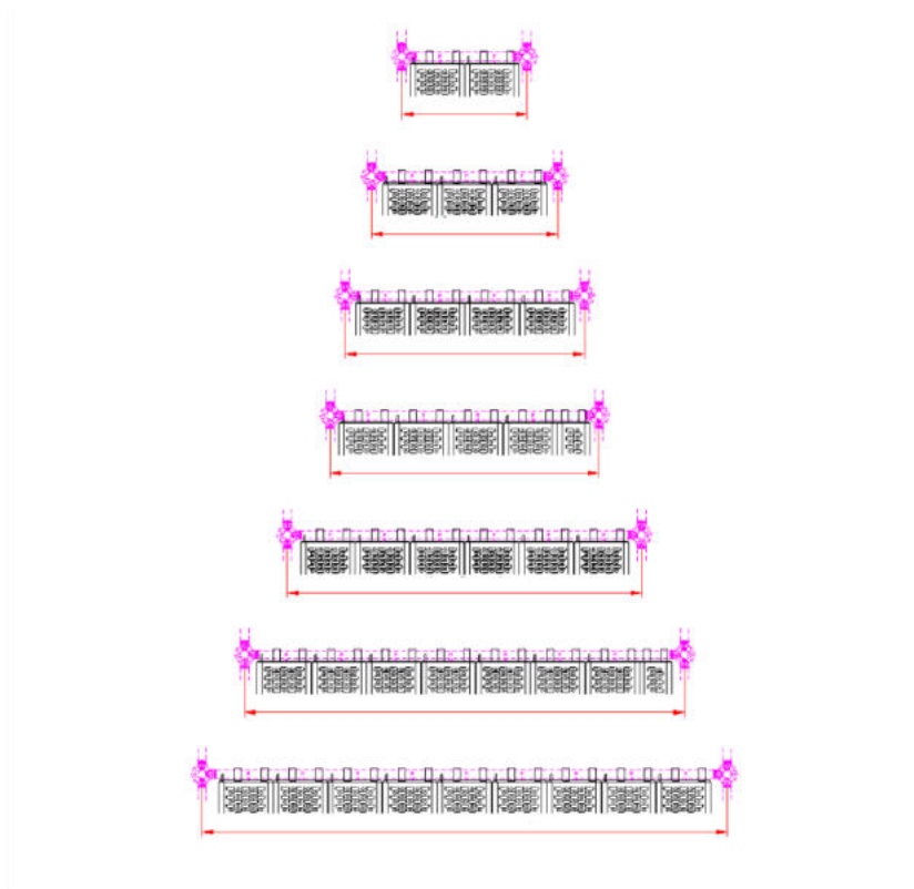
Figure 5.3 : Combinaison de planches en acier
