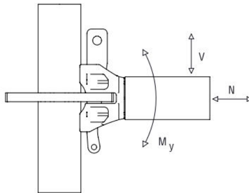
Figure 2.4 : Nœud fixé
